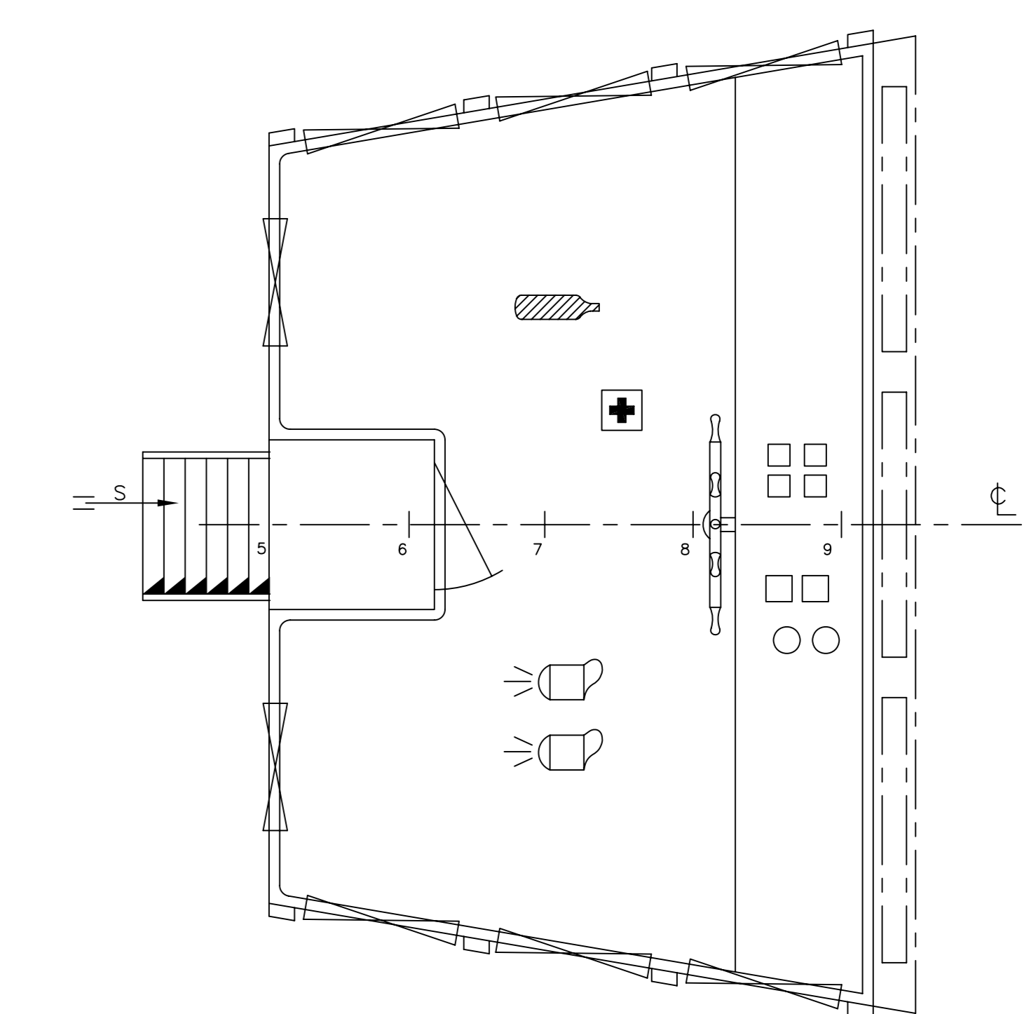
PLANTA DA CASA DO LEME
