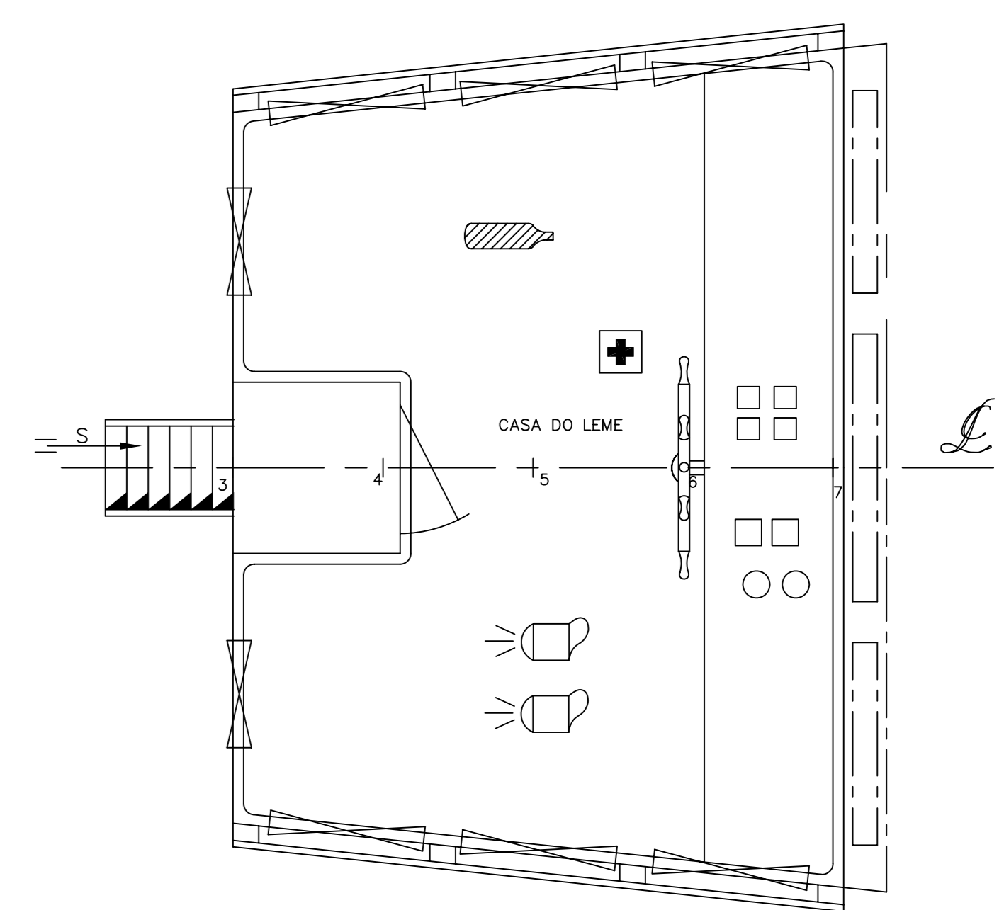
PLANTA DA CASA DO LEME
